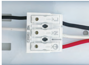
-端子台- WAGO製
